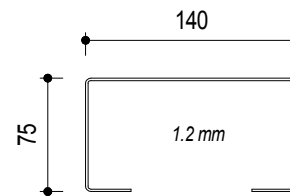
JUMBO STUD.
