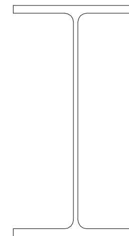
310 U.B. 40.4
